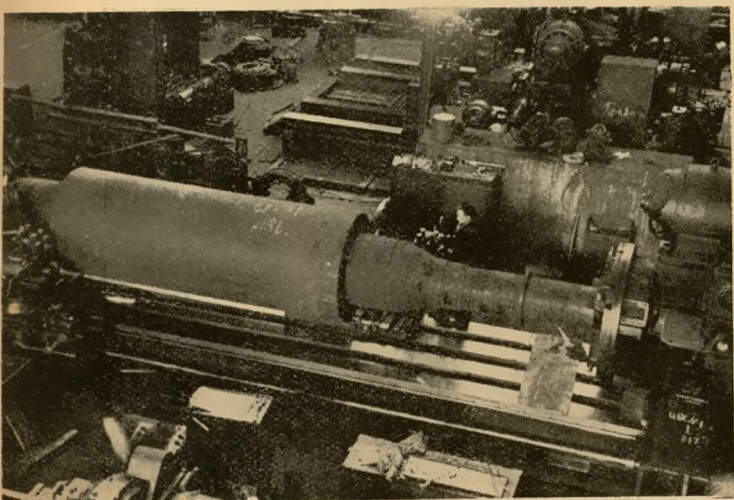
W dziale turbogeneratorów. Obróbka wału turbogenera- tora o mocy 50 tys. kilowatów.
