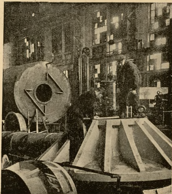
Zakłady produkują turbogeneratory dla Skiwskiej elektrowni państwowej, moc 30.000 KW. Na zdjęciu kontrola części turbogeneratorskiej.
