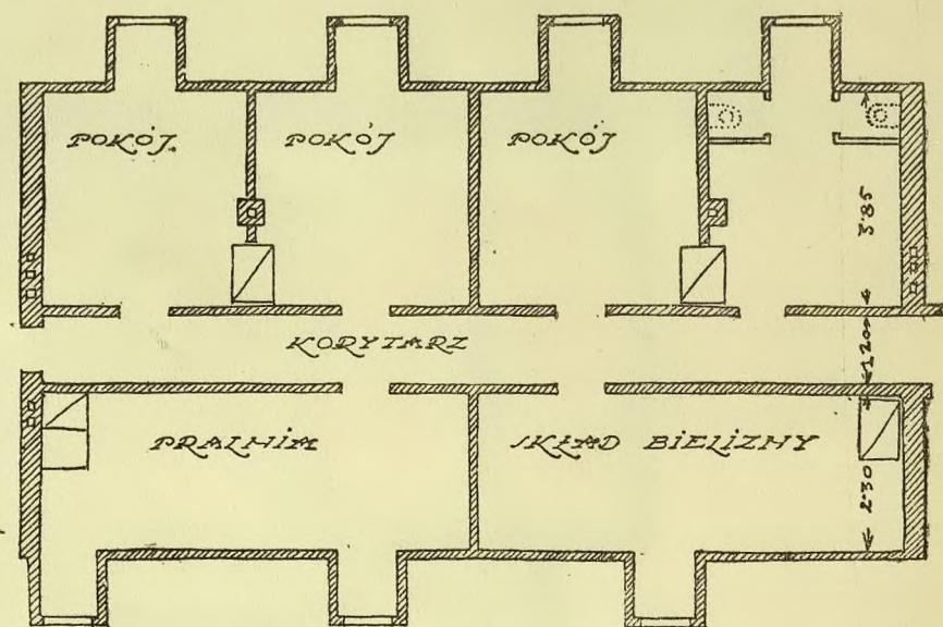
RZUT GÓRKI
