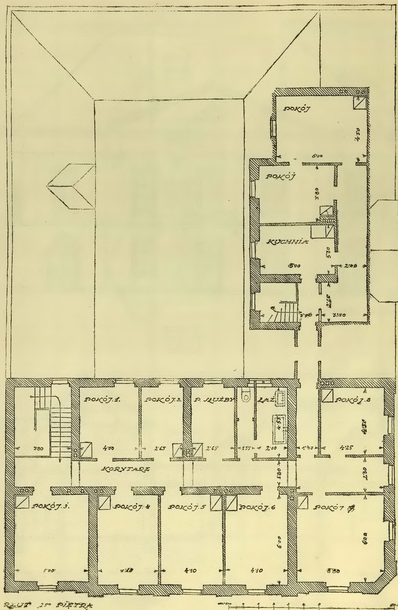
STEFAN STĘPKOWSKI. HOTEL Z ZAJAZDEM.
