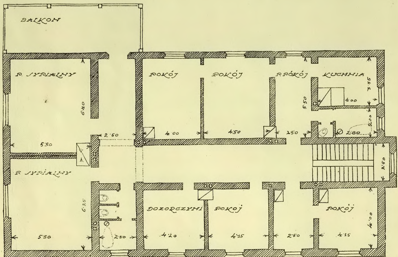
RZUT 1 o PIĘTRA DLA MĘŻCZYZN
