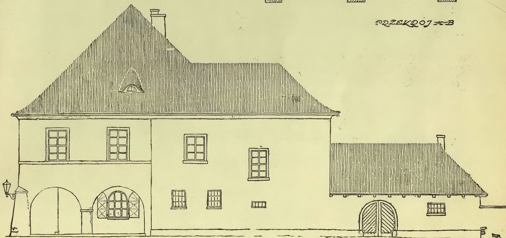
WIDOK BOCZNY
