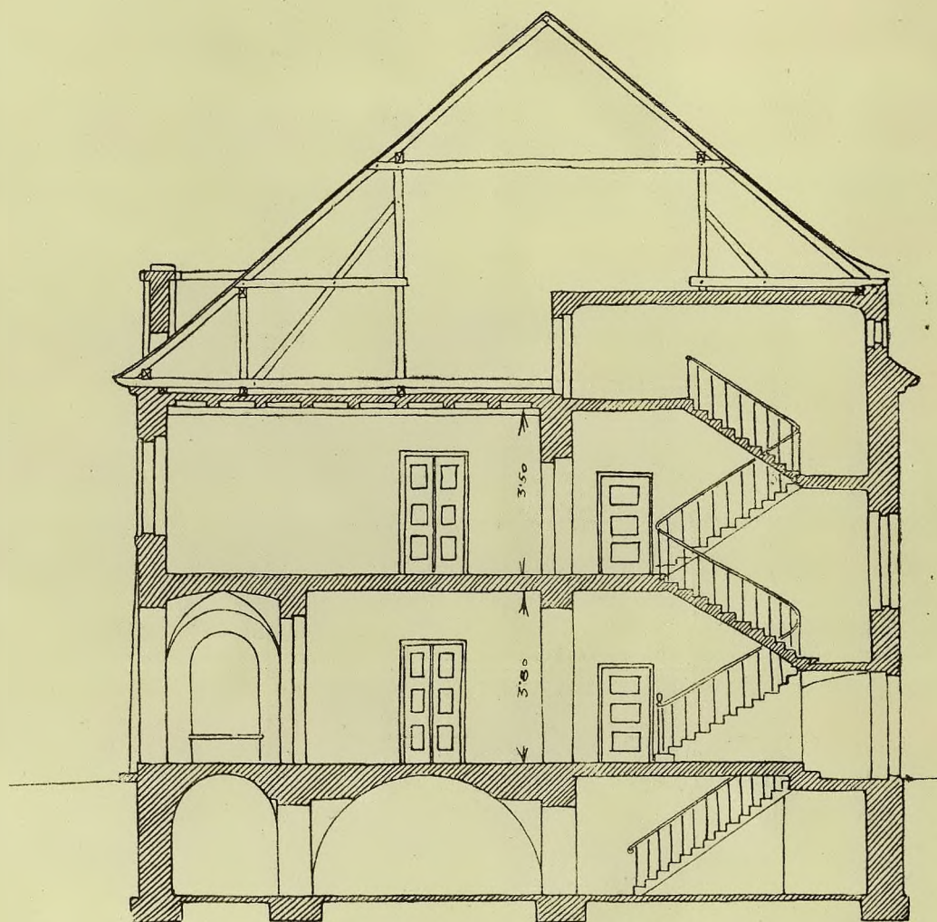
PRZĘKROJ A-B
