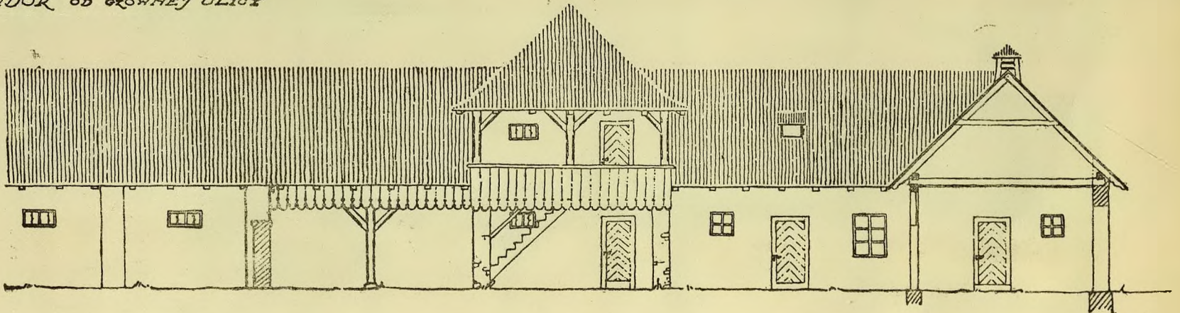
WIDOK OD GŁÓWNEJ ULICY
