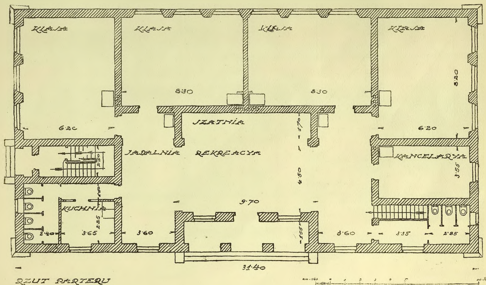
WITOLD MAŁKOWSKI. SZKOŁA LUDOWA CZTEROKLASOWA.
