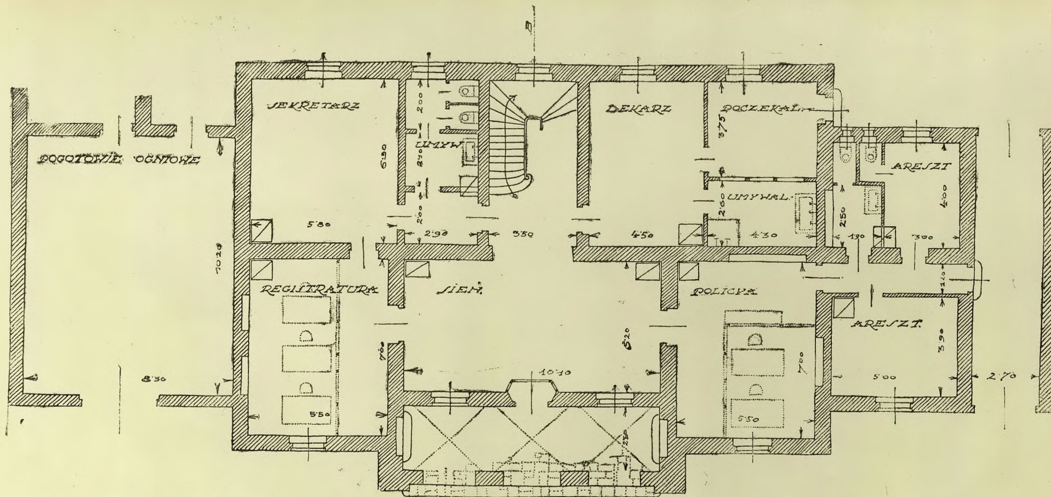
RZUT PARTERU
