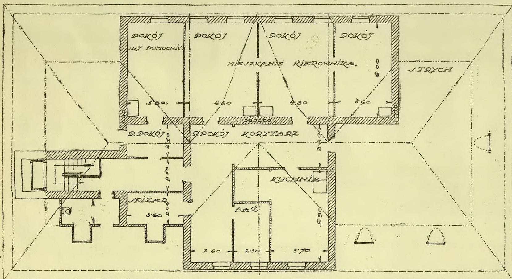
RZUT GÓRNY
