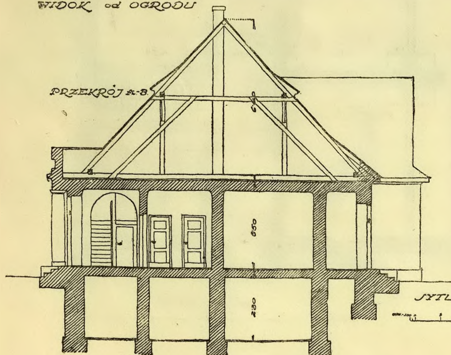
JÓZEF POKUTYŃSKI. DOM MIESZKALNY NAUCZYCIELI LUDOWYCH.
