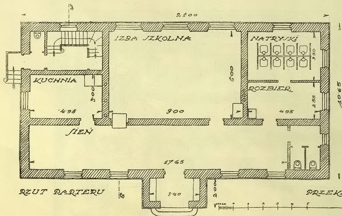
KAROL STRYJEŃSKI. SZKOŁA LUDOWA JEDNOKLASOWA.
