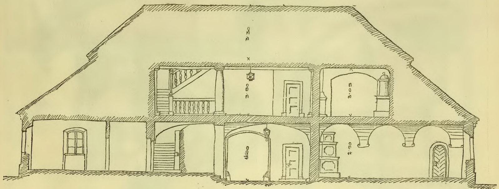
PRZĘKROJ PODRZECZNY
