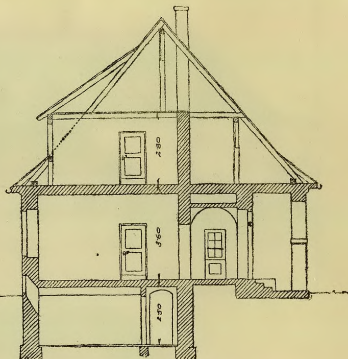
PRZĘKROJ A-B
