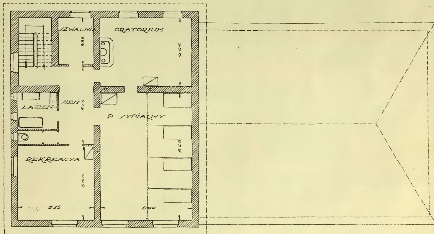
RZUT 1 o PIĘTRA
