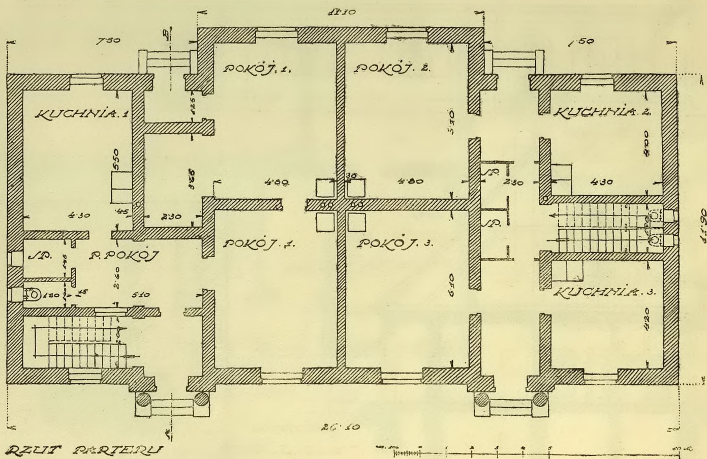
JÓZEF POKUTYŃSKI. DOM MIESZKALNY NAUCZYCIELI LUDOWYCH.
