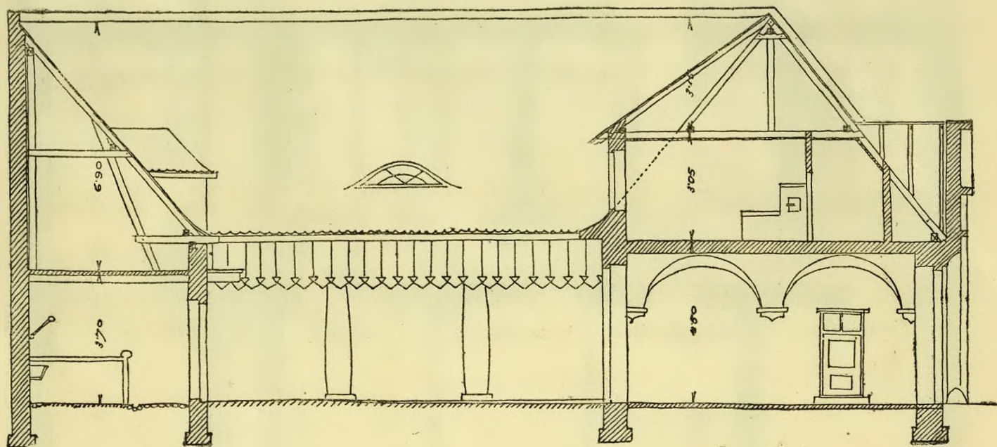
PRZEMKÓJ C-D
