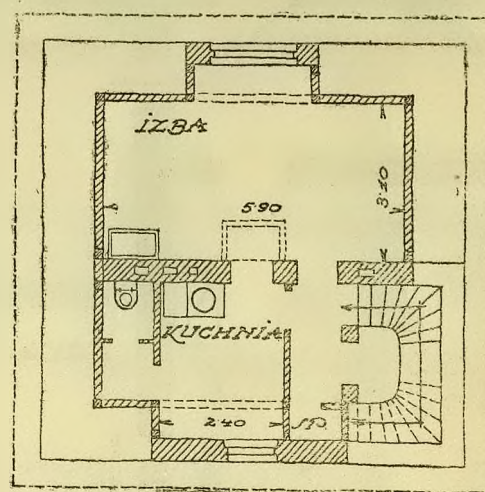
RZUT GÓRKI
