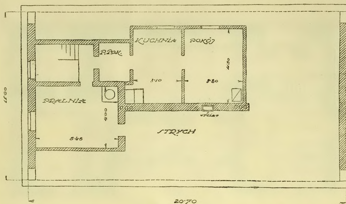
RZUT GÓRNY
