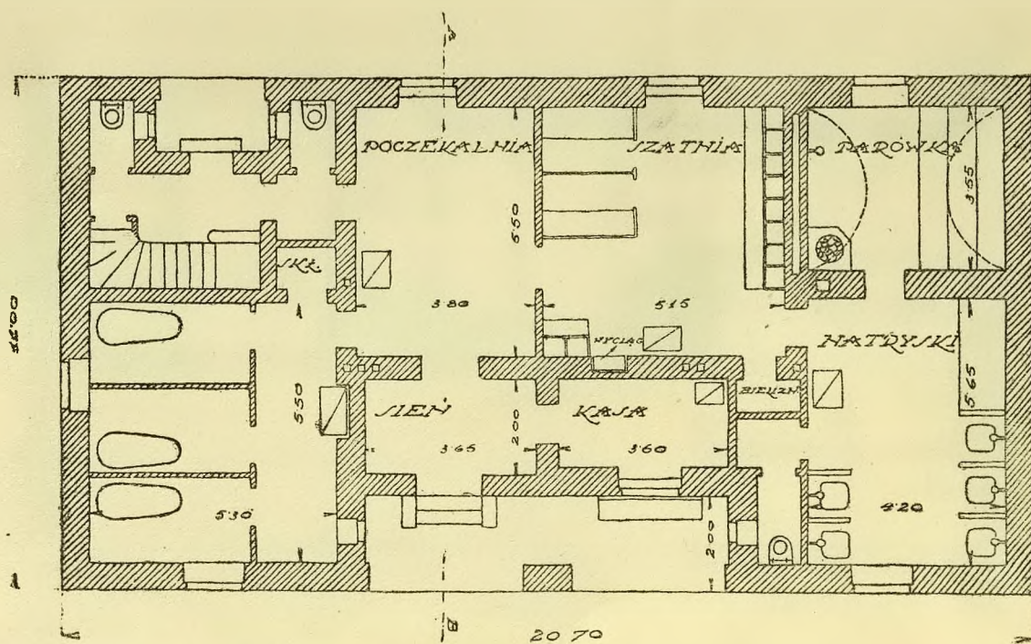
REUT PARTERU
