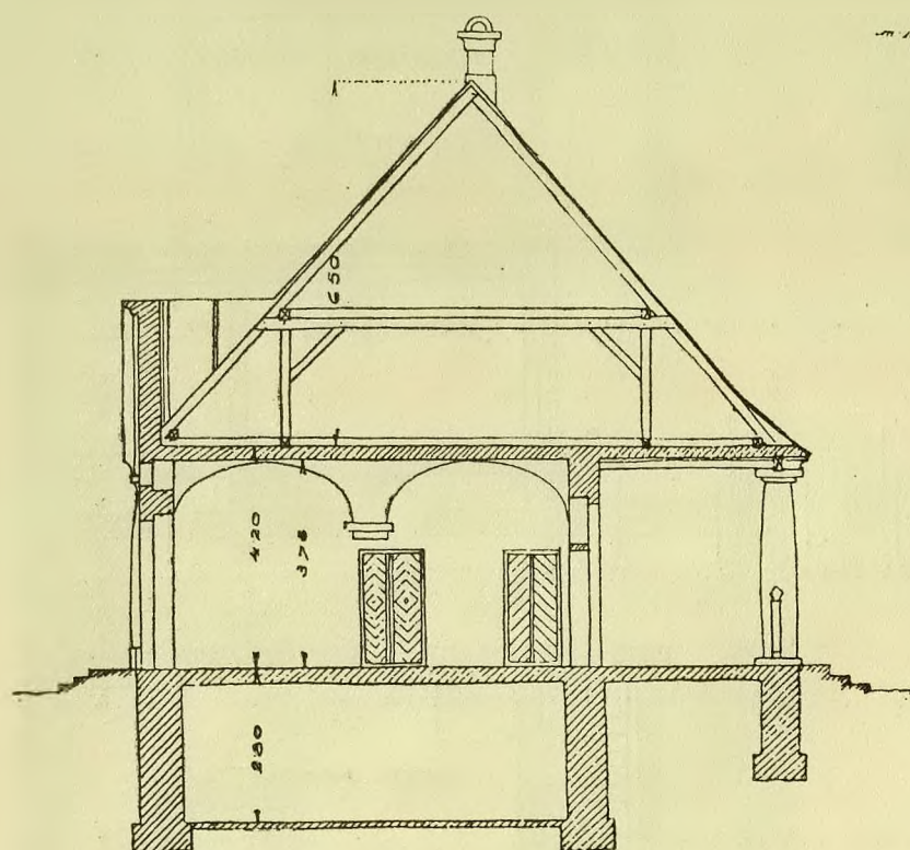
PRZĘKROJ A-B
