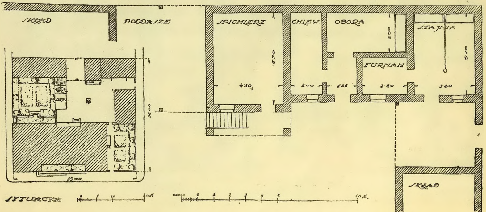
ZYGMUNT HARLAND. DOM LUDOWY, MNIEJSZY.
