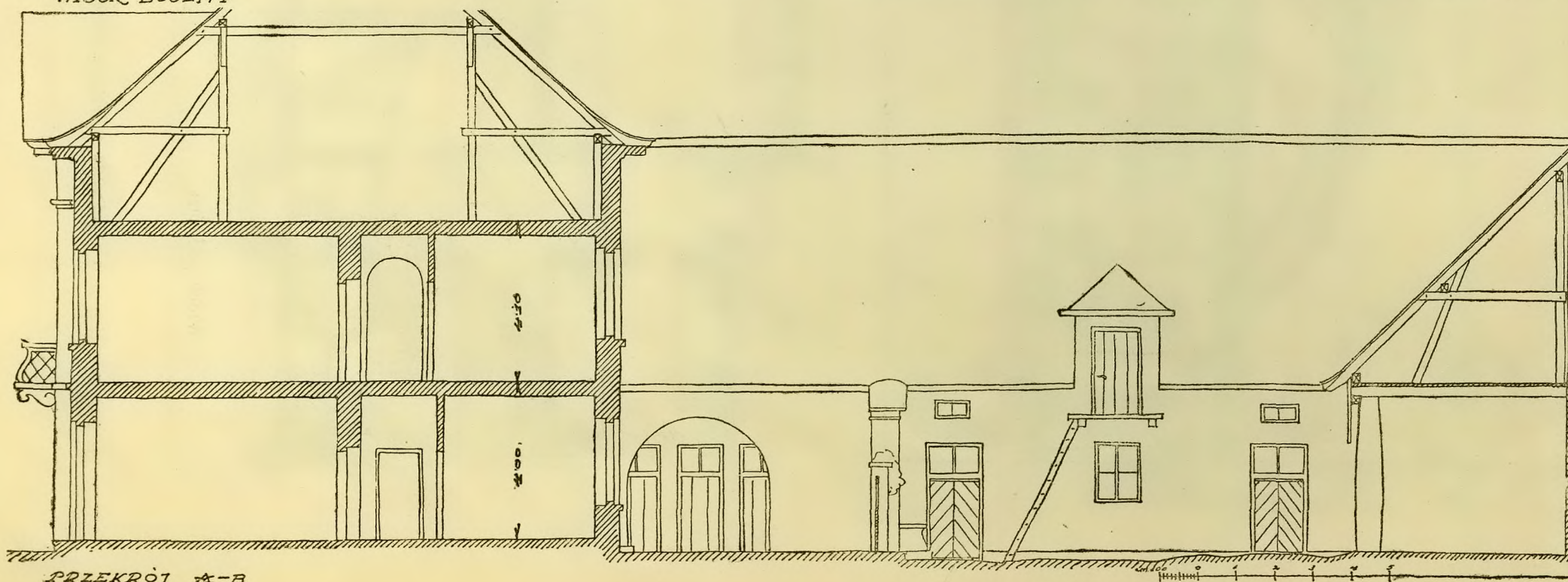
PRZEMKÓJ A-B
