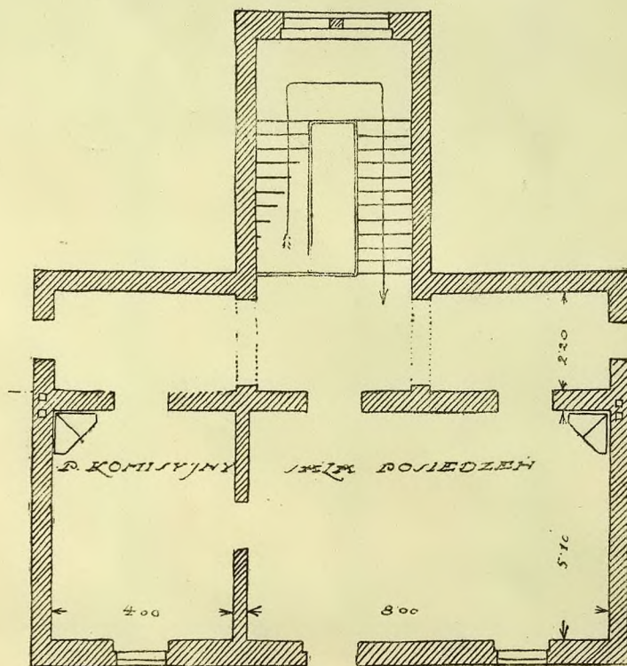
RZUT GÓRNY
