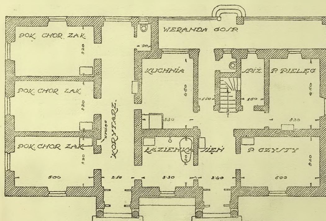
RZUT PARTERU
