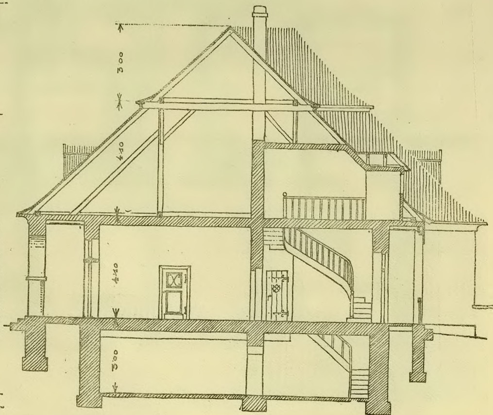
PRZEKRÓJ A-B
