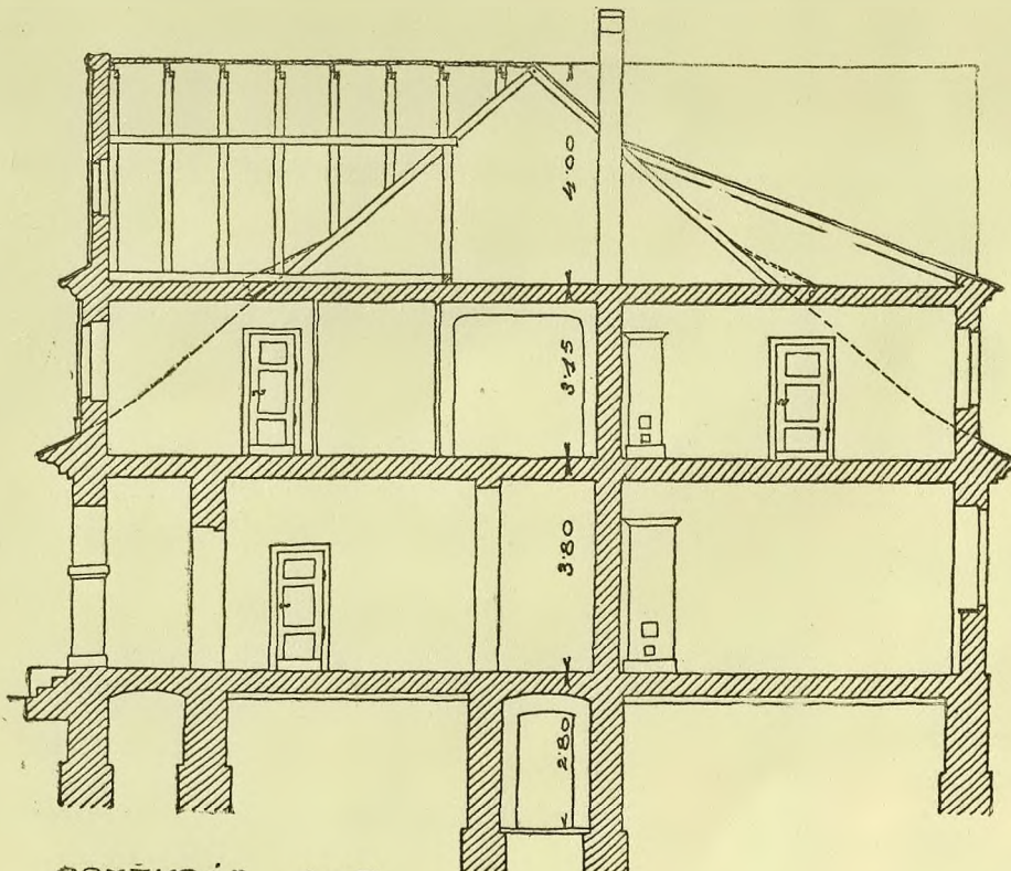
PRZĘKRÓJ A-B
