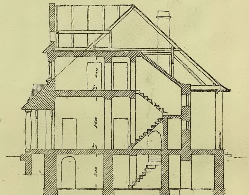
PRZEKROJ A-B
