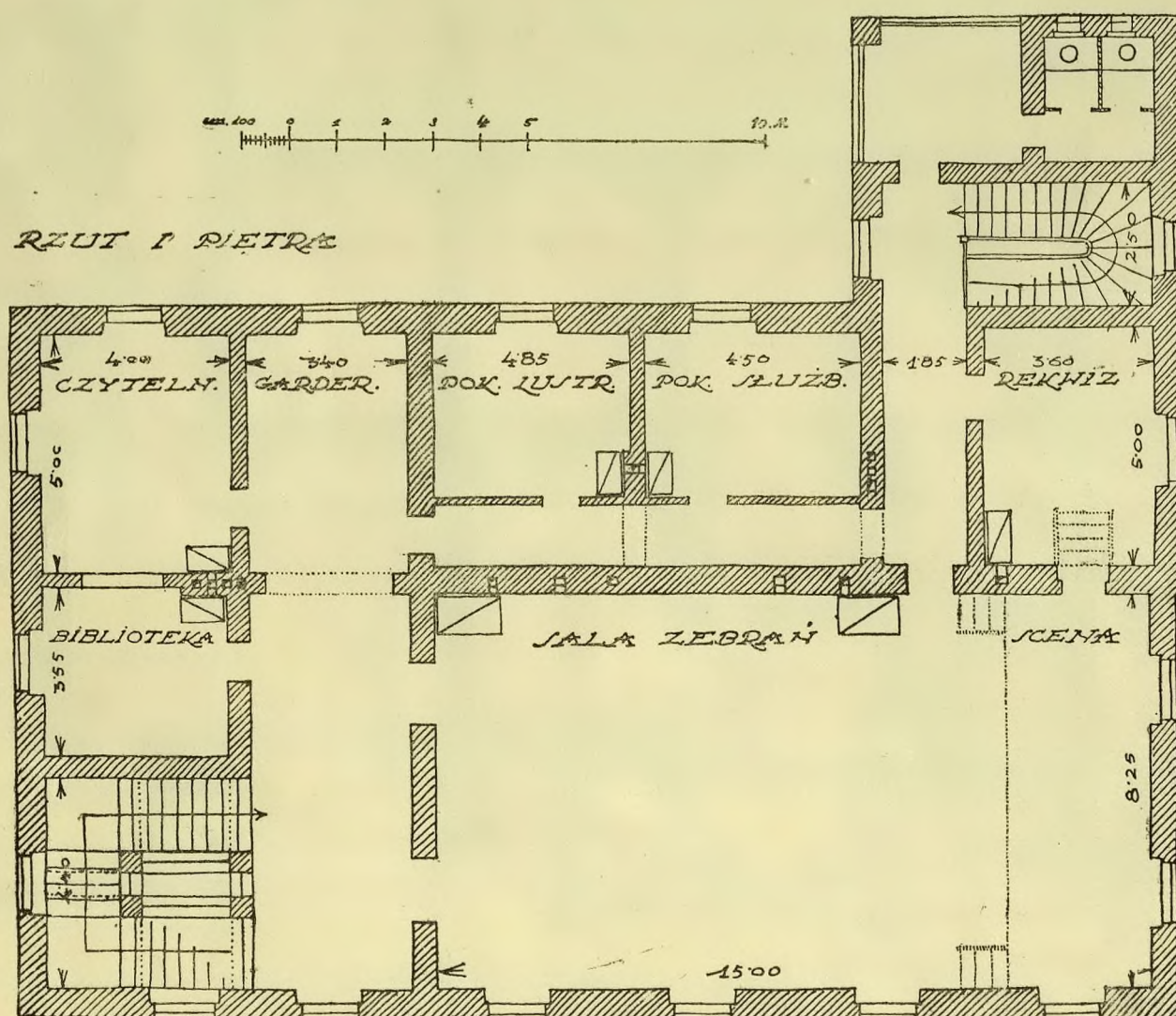
ZYGMUNT HARLAND. DOM LUDOWY, WIĘKSZY.
