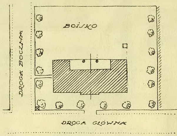
SYTUACJA
