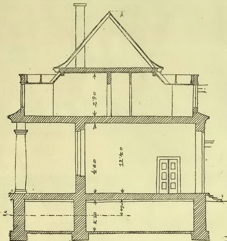
PRZEMKÓJ A-B
