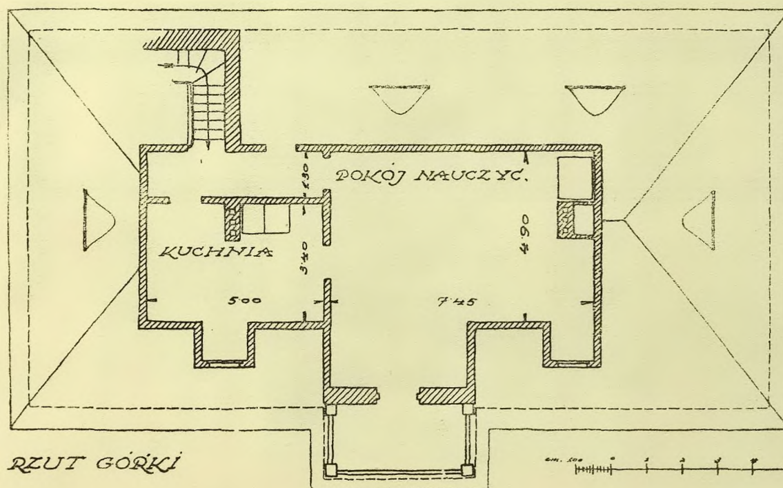
KAROL STRYJEŃSKI. SZKOŁA LUDOWA JEDNOKLASOWA.
