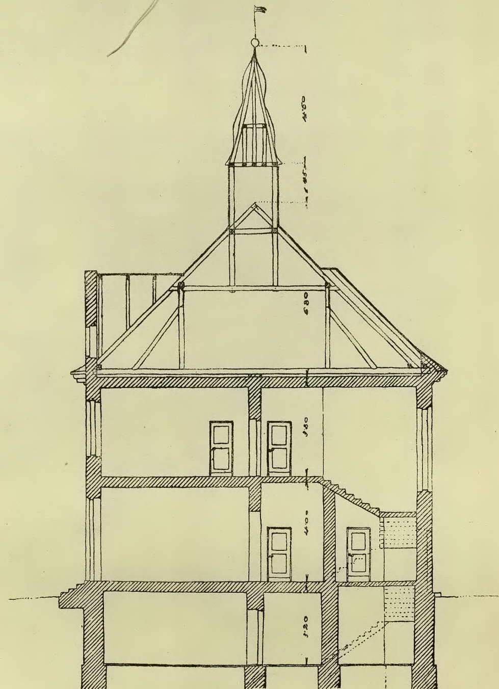
PRZĘKROJ A-B
