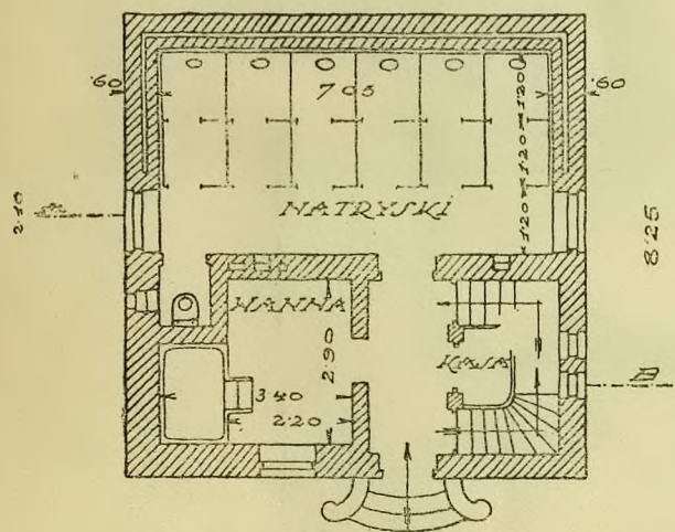
RZUT PARTERU
