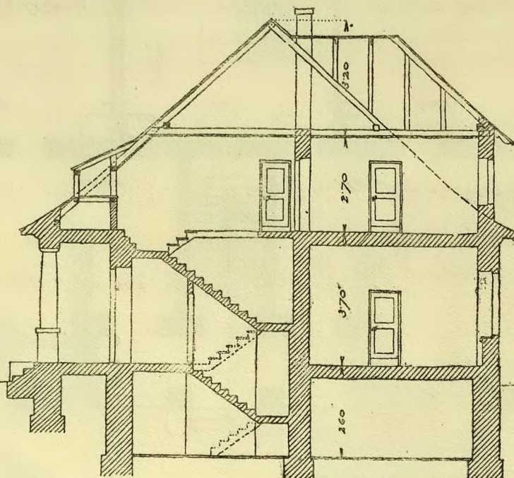
PRZEMKÓJ A-B
