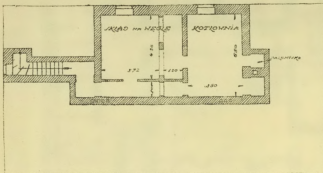
RZUT PIWNIC
