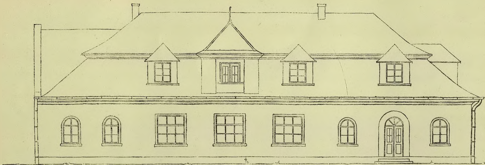
WIDOK FRONTOWY
