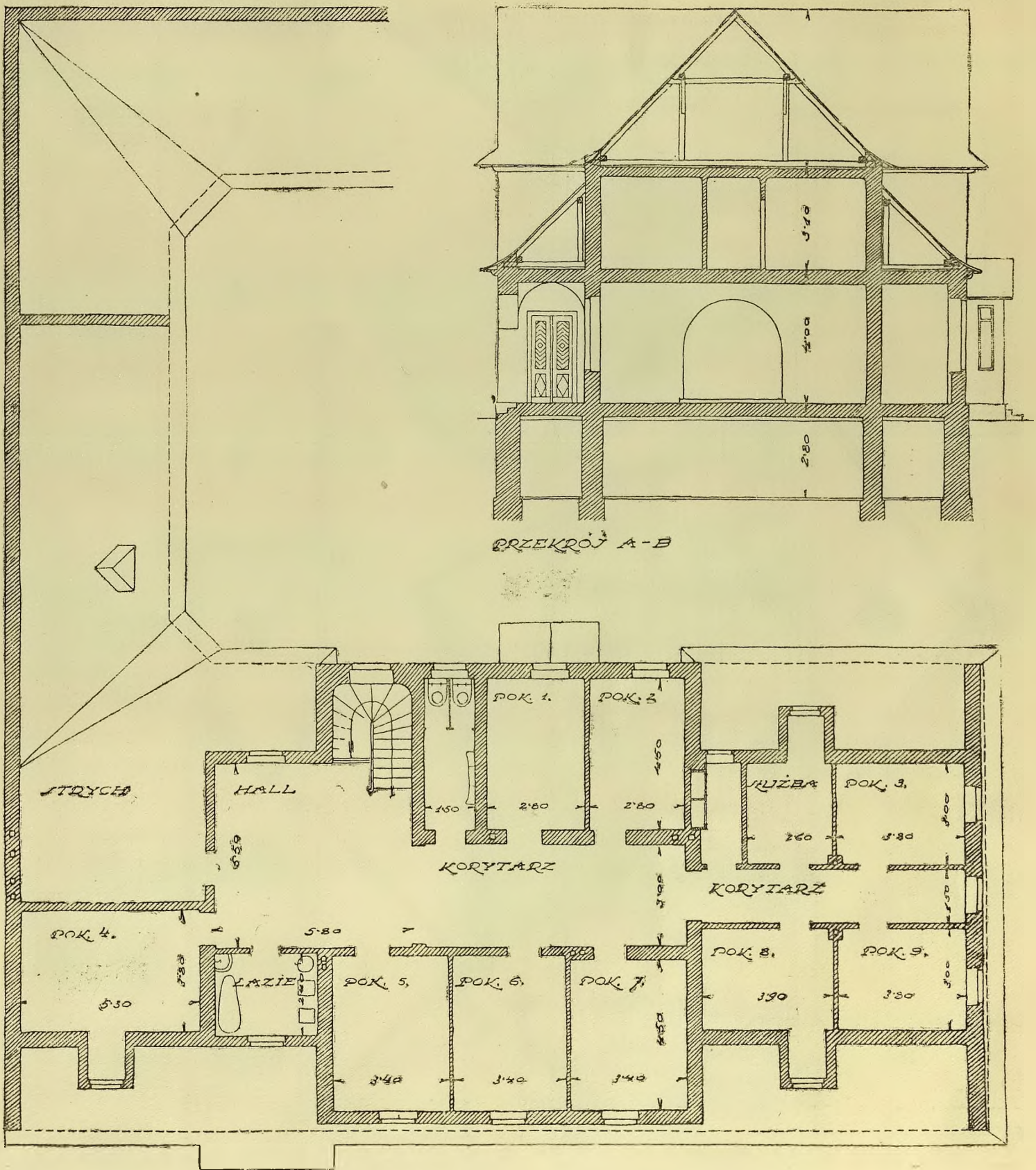
RZUT GÓRNY
