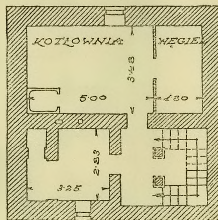
RZUT PIWNIC
