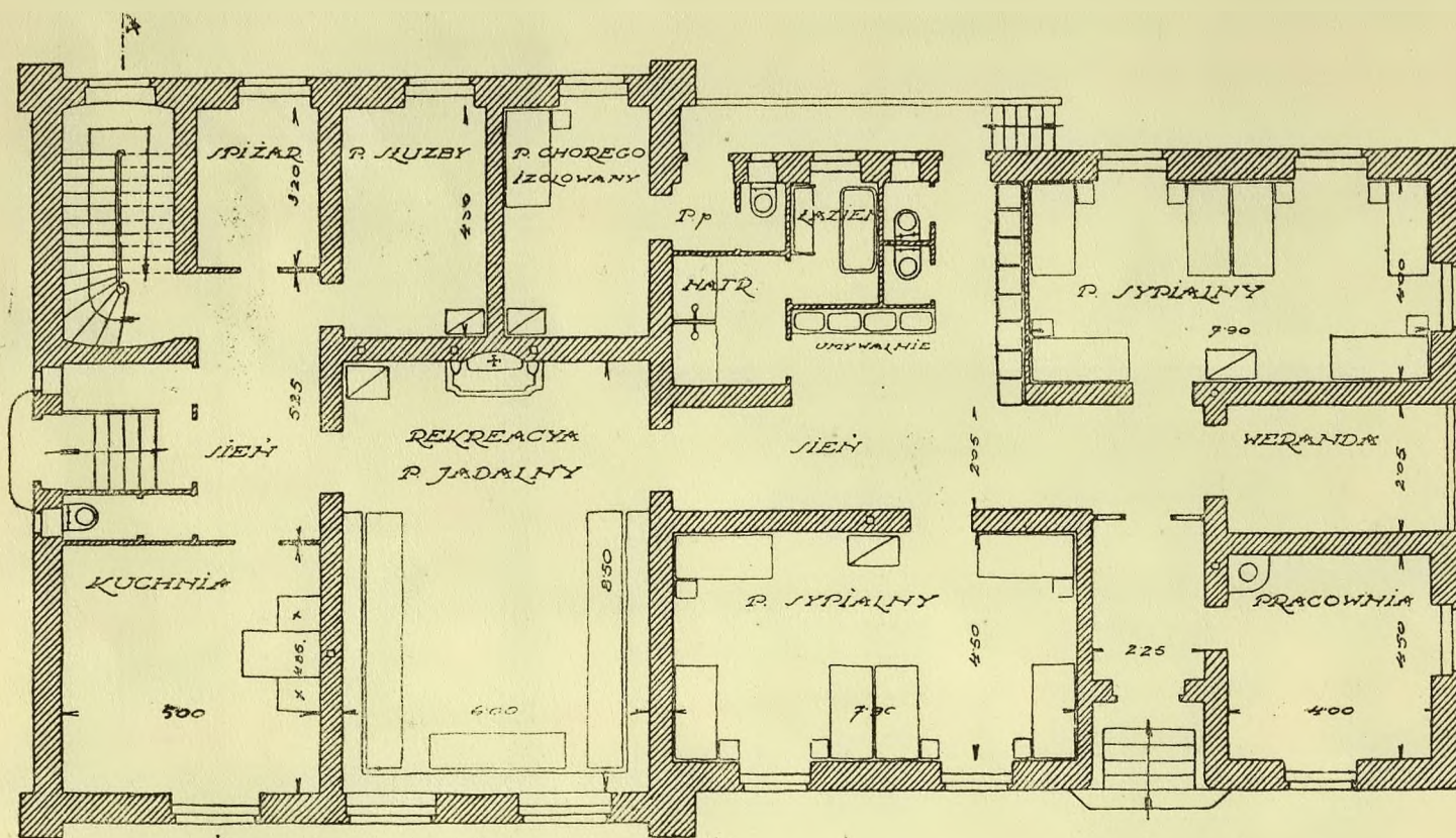
RZUT PARTERU
