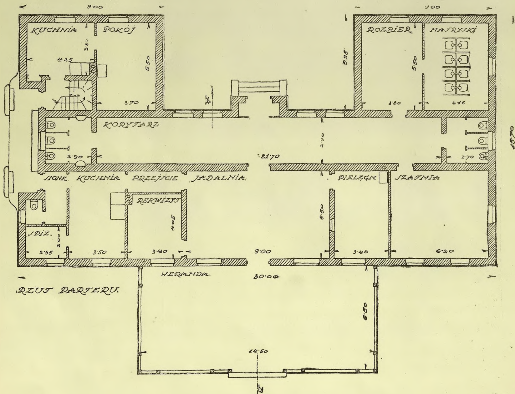
FRANCISZEK MACZYŃSKI. PÓŁKOLONIA.
