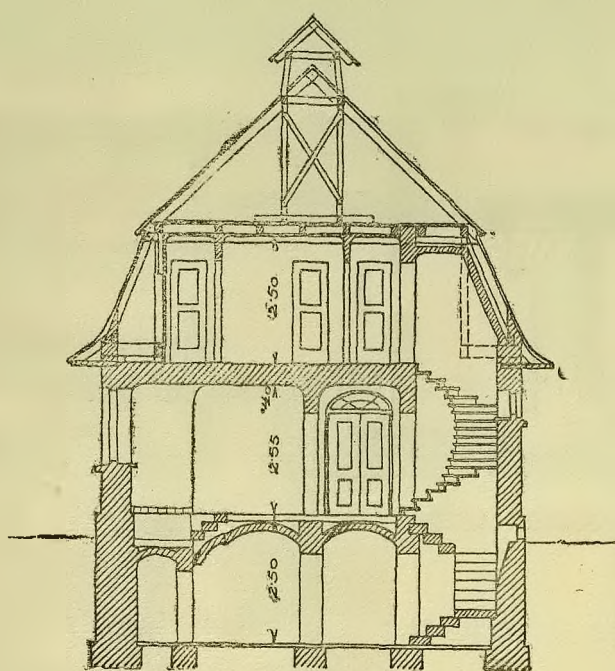
PRZĘKROJ A-B
