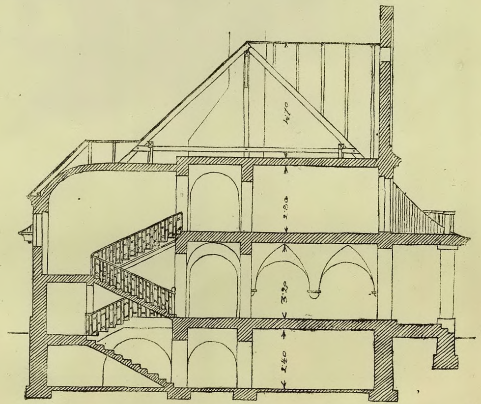
PRZESZKÓJ A-B
