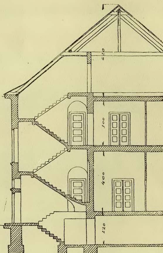
PRZĘKRÓJ A-B
