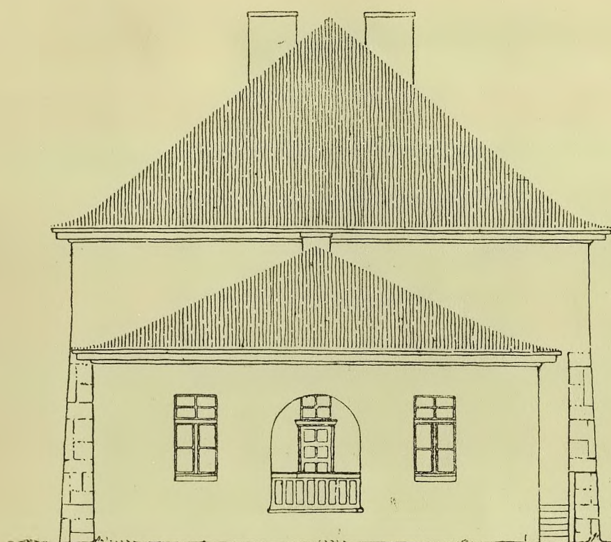
WIDOK BOCZNY
