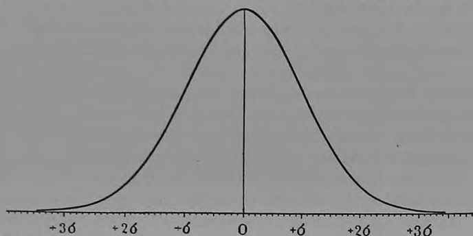
Fig. 1. Die sog. „ideale Variationskurve“, welche die Verteilung der Varianten einer ganz symmetrischen, „idealen“ Variationsreihe illustriert. Auf der Grundlinie sind zu beiden Seiten des Mittelwerts die Abweichungen markiert, 0 = Mittel, \sigma = Standardabweichung.
