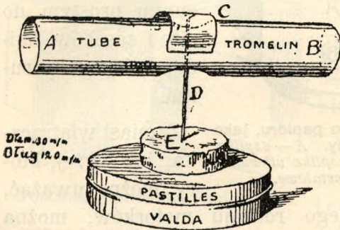
Tuba Tromelina. C—siodelko przyklejone z metalu. E—korek, w którym utkwiona szpilka.
