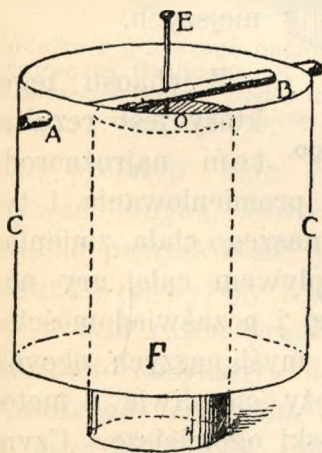
Zasadniczy typ motoru (wiatraczka) fluidycznego. AB — słomka, EO — szpilka, F — szklane naczynie, na powierzchni którego opiera się ostrze szpilki O .
