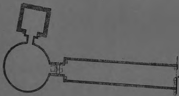
8. u. 9. Das sog. Schatzhaus des Atreus. Durchschnitt und Grundriss.
